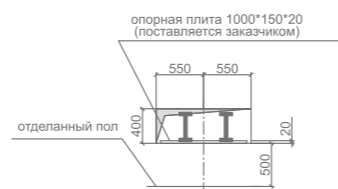
A-A грузоподъёмность проёма
