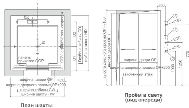
План шахты
