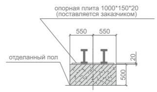
B-B грузоподъёмность пирса
