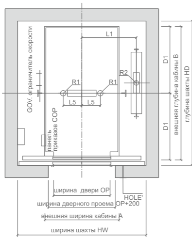
План шахты
