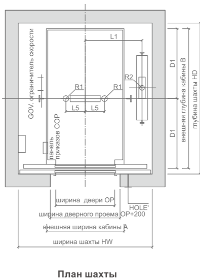
План шахты
