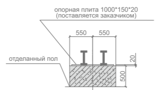
B-B грузоподъемность пирса
