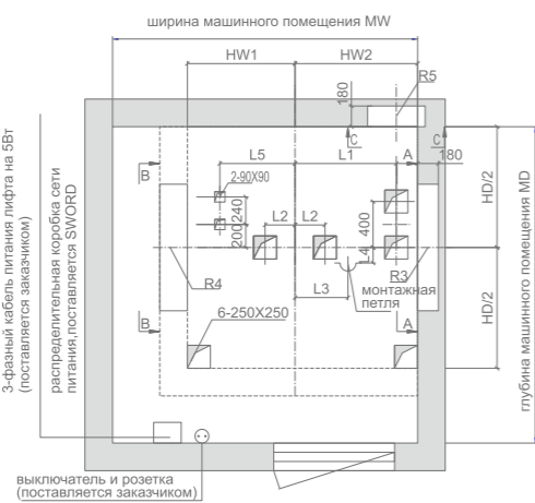
план устройства отверстий для машинного помещения
